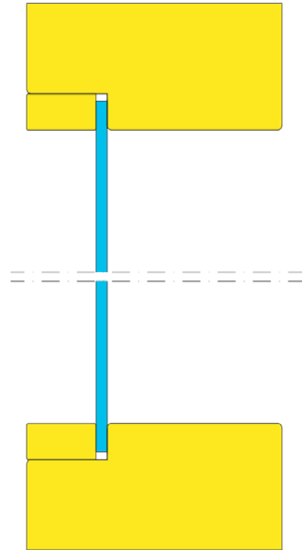
Sisäikkuna 1K-lasituksella
